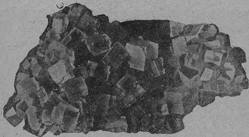
Плавиково шпато. Кристаллы.
